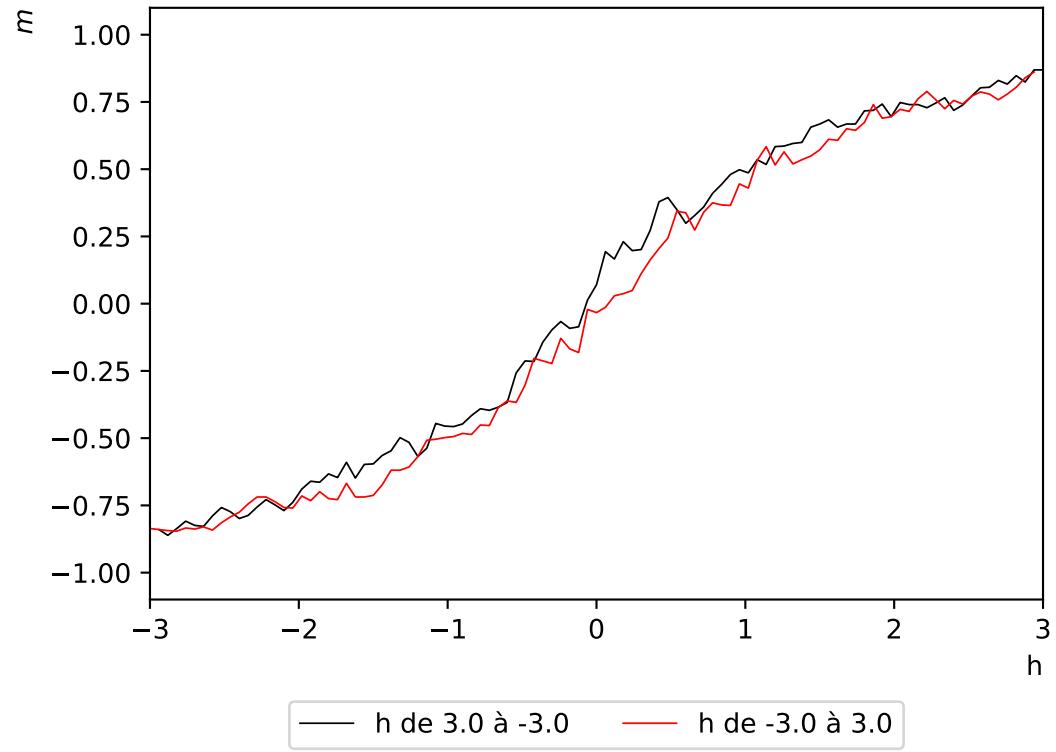
Hystérésis de l'aimantation - réseau de taille L=32 - champ magnétique d'amplitude h=3 à T=5.0
